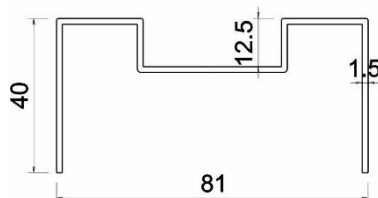
Code: PDA1920 L : 6.0m G AL : 2.14kg/m
