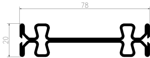
Code: PDA1882CA L : 6.0m G : 3.16kg/m
